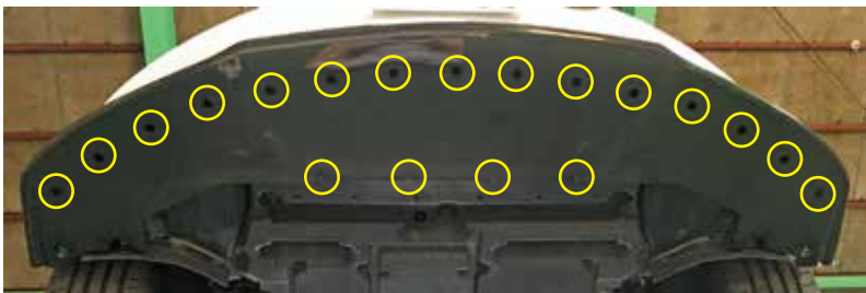
トラスタッピングビス取り付け位置
