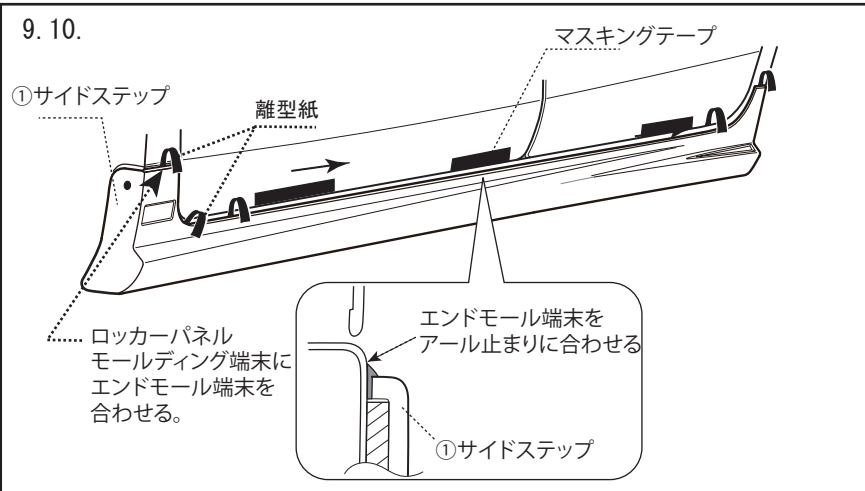
取付断面図
