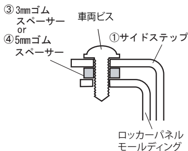
取付断面図
