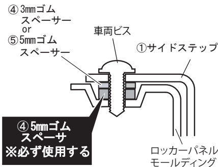
取付断面図
