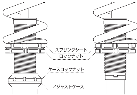
全長調整式ネジ式車高調整
